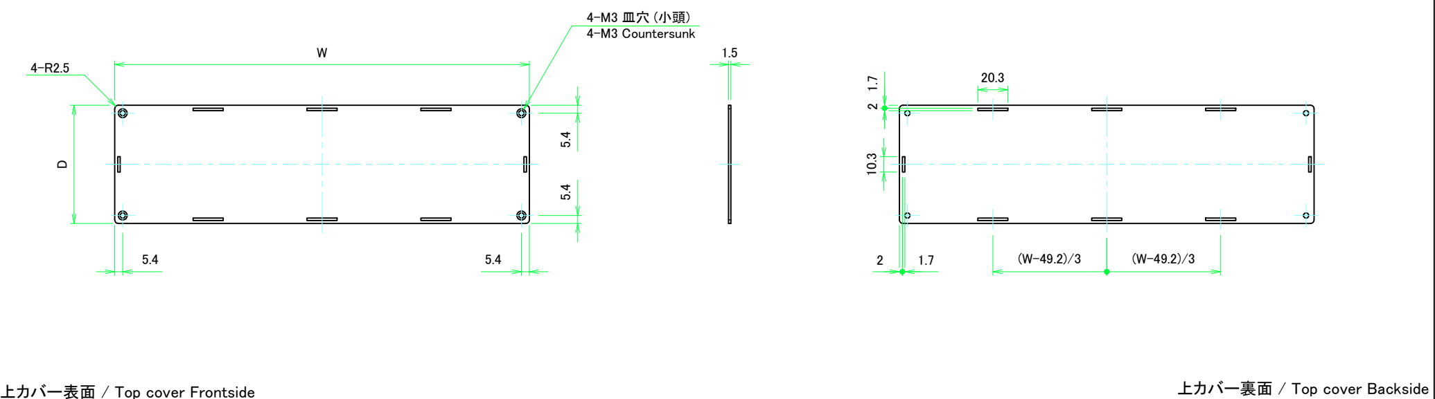
上カバー表面 / Top cover Frontside
