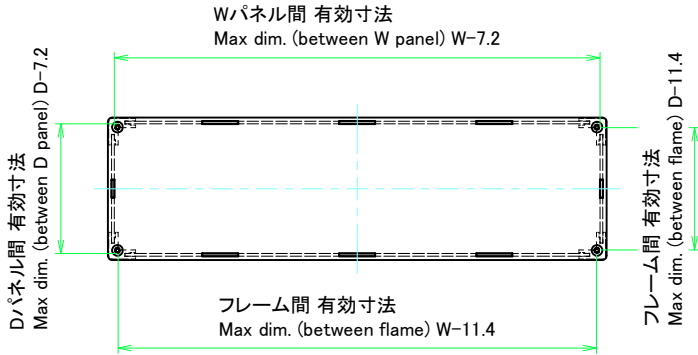
下カバー / Bottom cover
